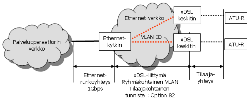
Kuva 2. xDSL-Ethernet-operaattorituote, ryhmäkohtainen VLAN
