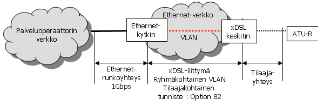
Kuva 3. xDSL-Ethernet-operaattorituote, tilaajakohtainen VLAN
